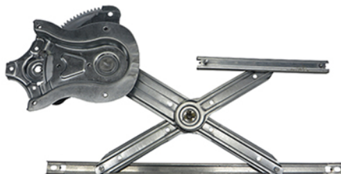
POWER WINDOW RIGHT ALZACRISTALLI ELETTRICO DX
